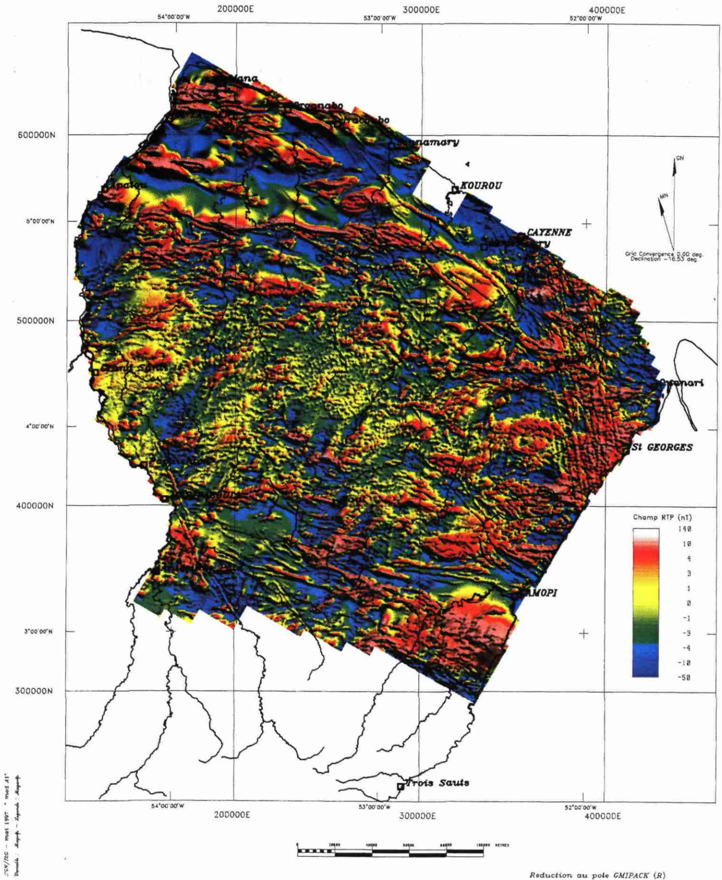
Fig. E - Magnétisme - Anomalie réduite au pôle.
