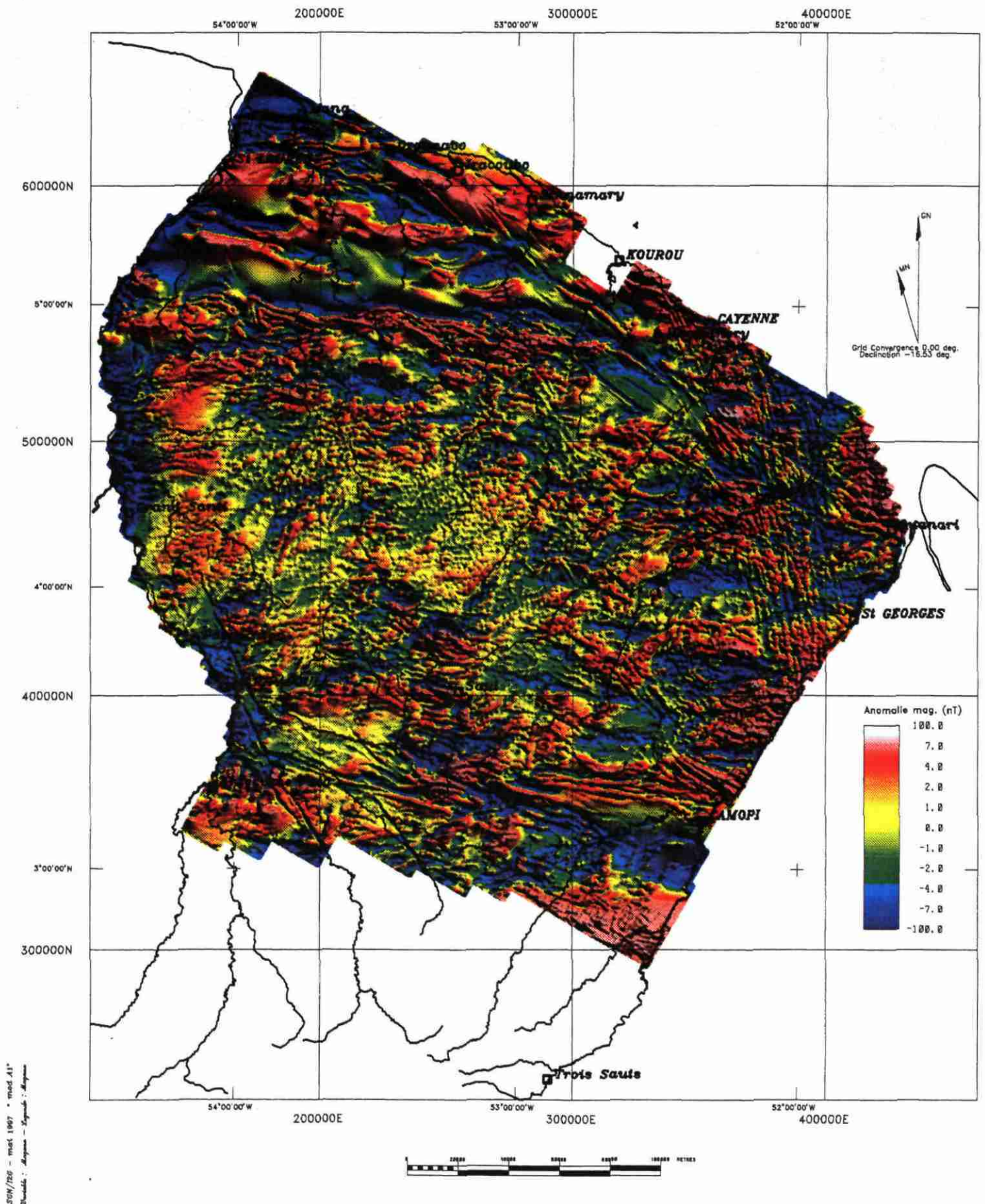
Fig. D - Magnétisme - Anomalie du champ total.
