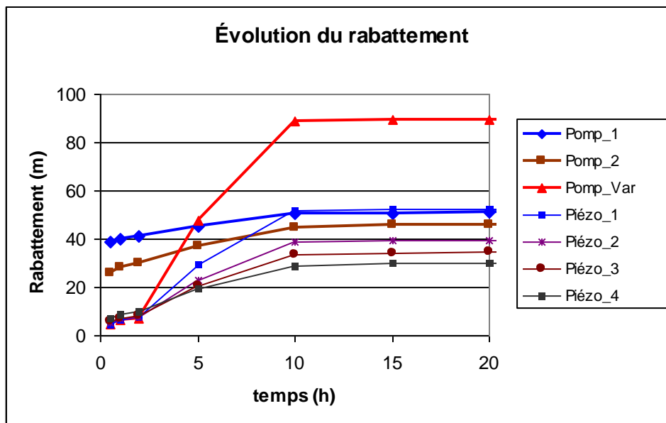
Figure 12 : Visualisation de l'évolution des rabattements calculés dans 3 puits et 4 piézomètres.
