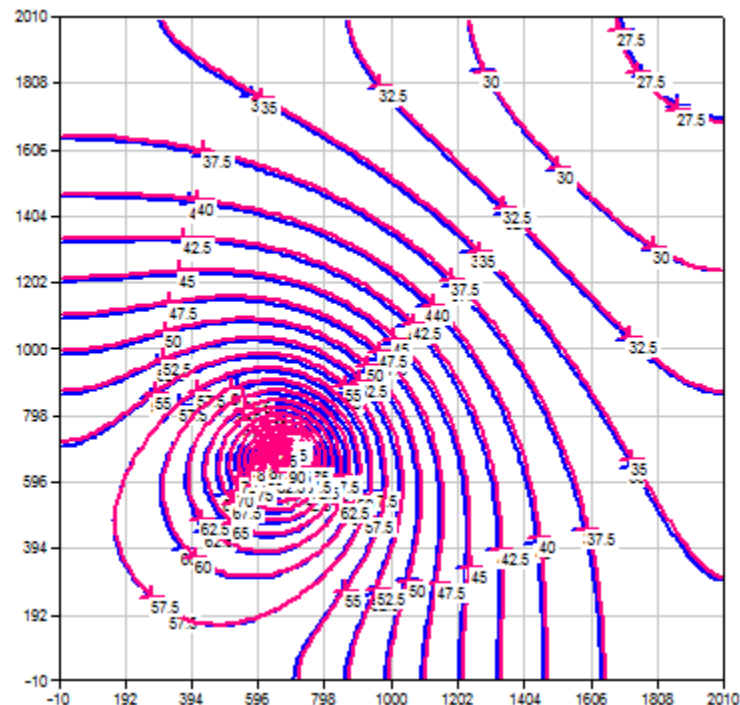
Figure 17 : Pompage au 1/3 inférieur d'un domaine carré dont les 4 limites sont étanches. Rabattement après 2 jours.
