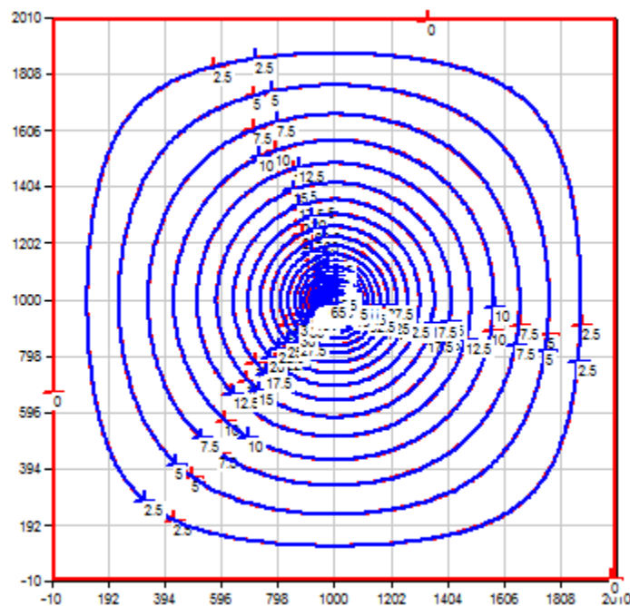
Figure 13 : Pompage au centre d'un domaine carré. Régime permanent.
