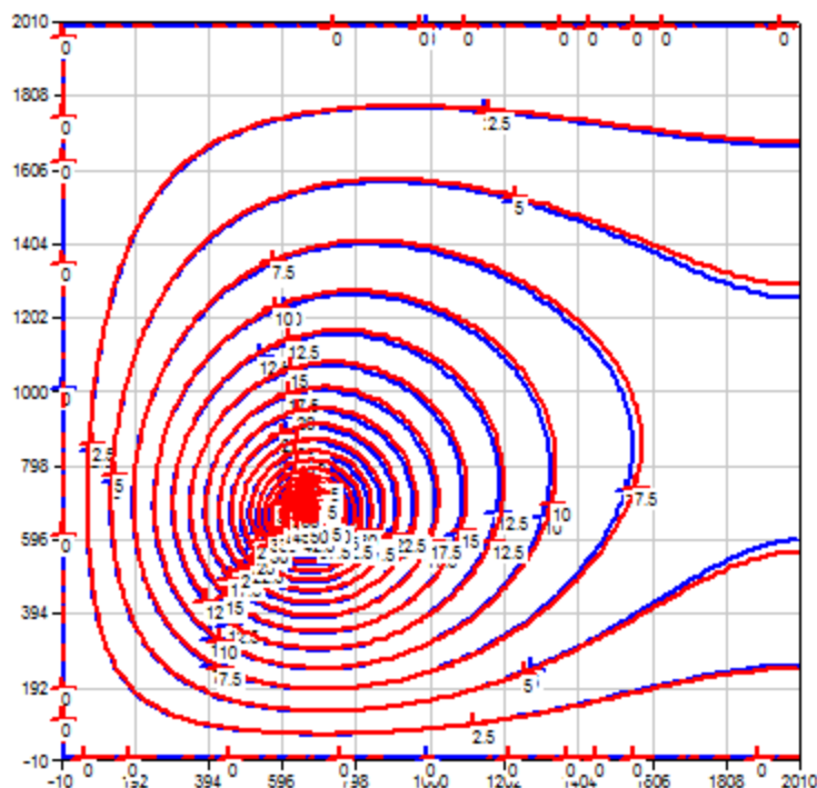
Figure 15 : Pompage au 1/3 inférieur d'un domaine carré dont 3 côtés sont à charge imposée. Rabattement après 50 jours.
