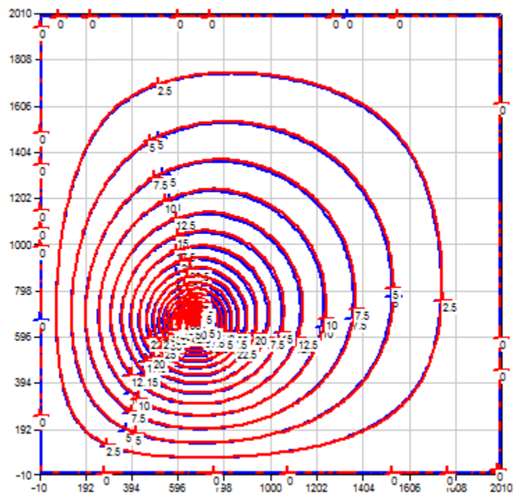
Figure 14 : Pompage au 1/3 inférieur d'un domaine carré. Rabattement après 50 jours.
