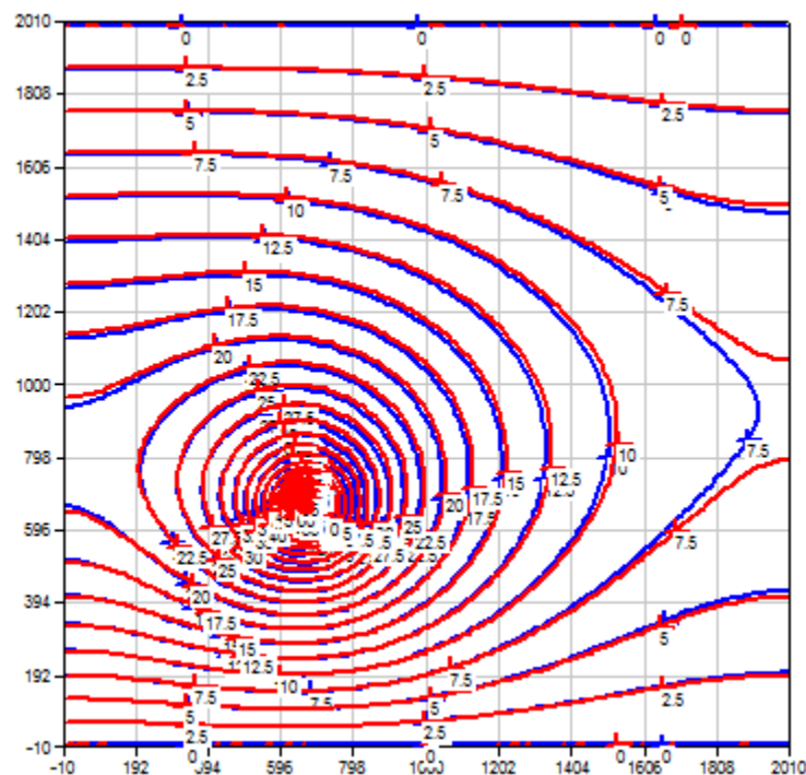
Figure 16 : Pompage au 1/3 inférieur d'un domaine carré dont les côtés parallèles sont des limites de même nature. Rabattement après 50 jours.
