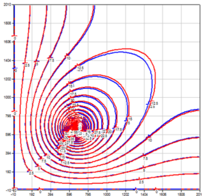
Figure 18 : Pompage au 1/3 inférieur d'un domaine carré dont les côtés parallèles sont des limites de nature opposée. Régime permanent.
