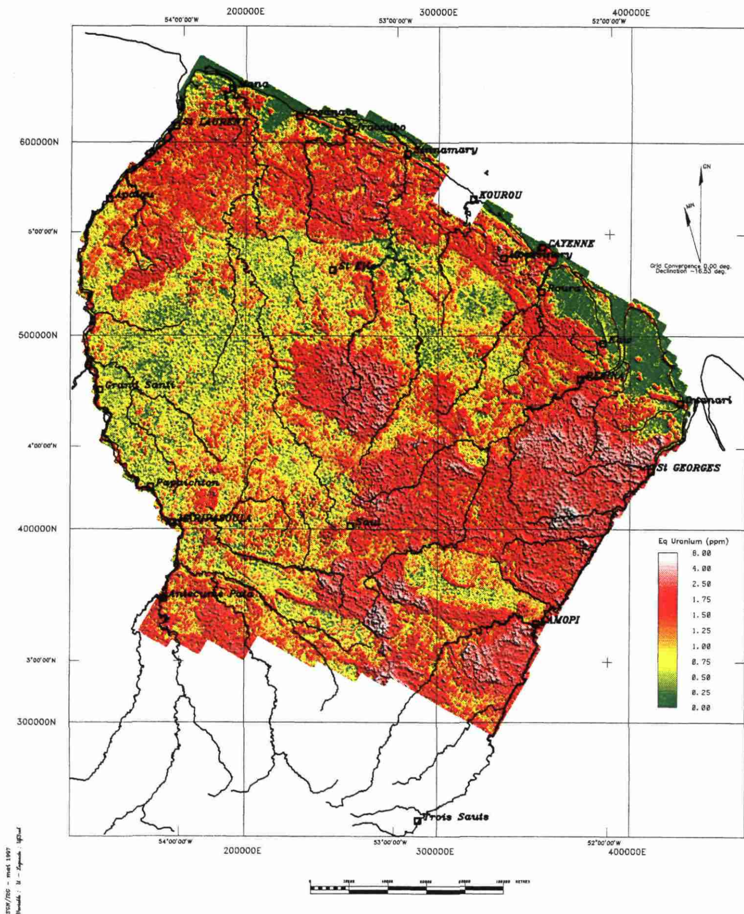
Fig. H - Radiométrie spectrale - Uranium.
