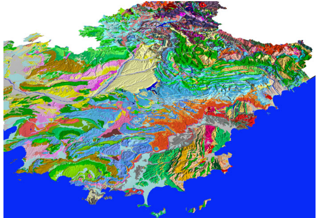
Carte géologique à 1/250 000 de la Région PACA
