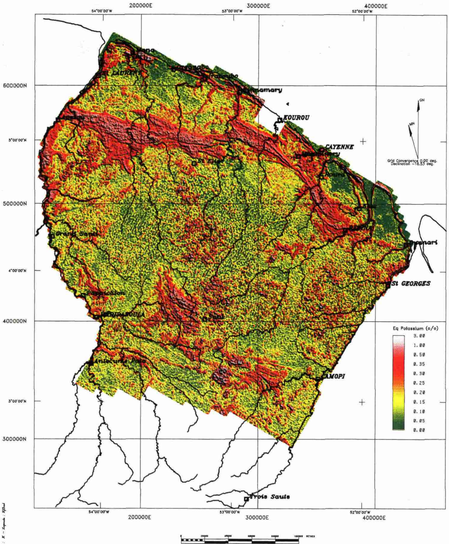
Fig. J - Radiométrie spectrale - Potassium.
