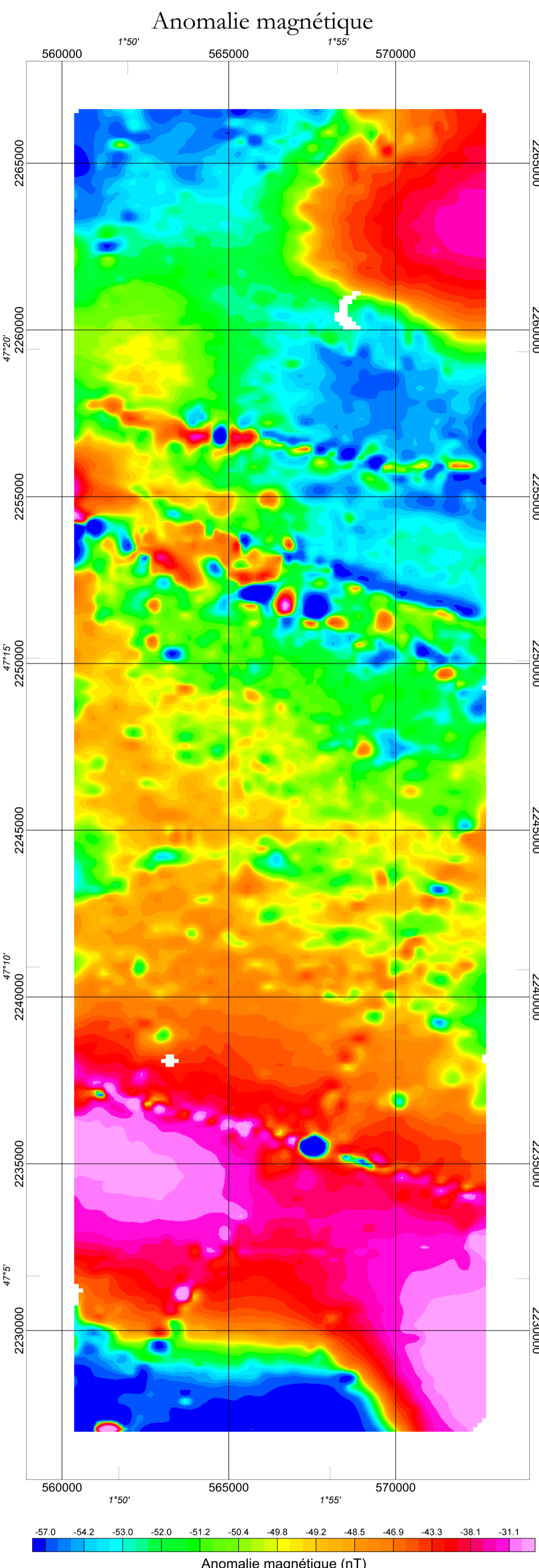
Anomalie magnétique (nT)
