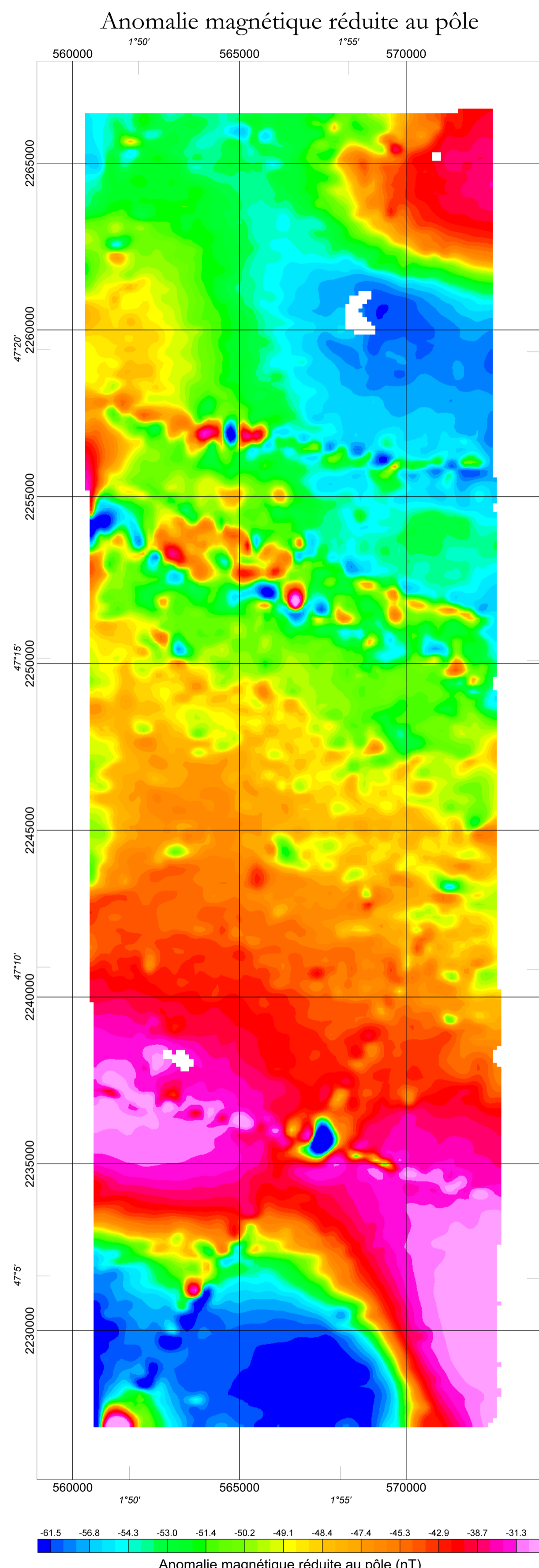
Anomalie magnétique réduite au pôle (nT)
