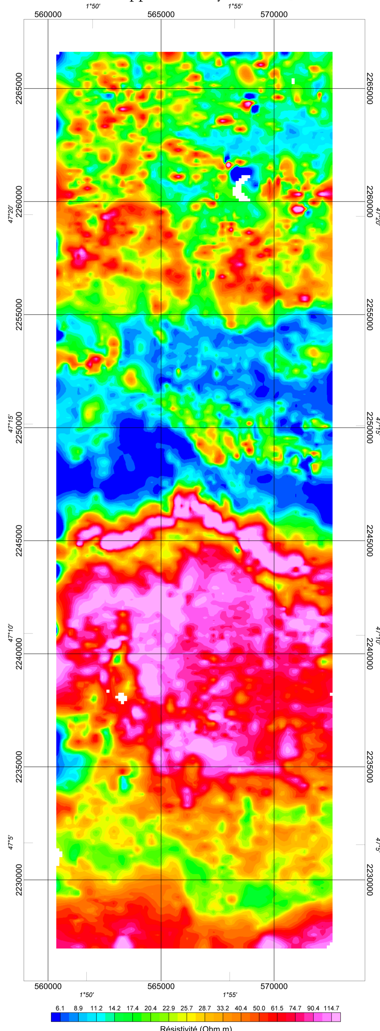
Résistivité apparente moyenne à 80/100 m
