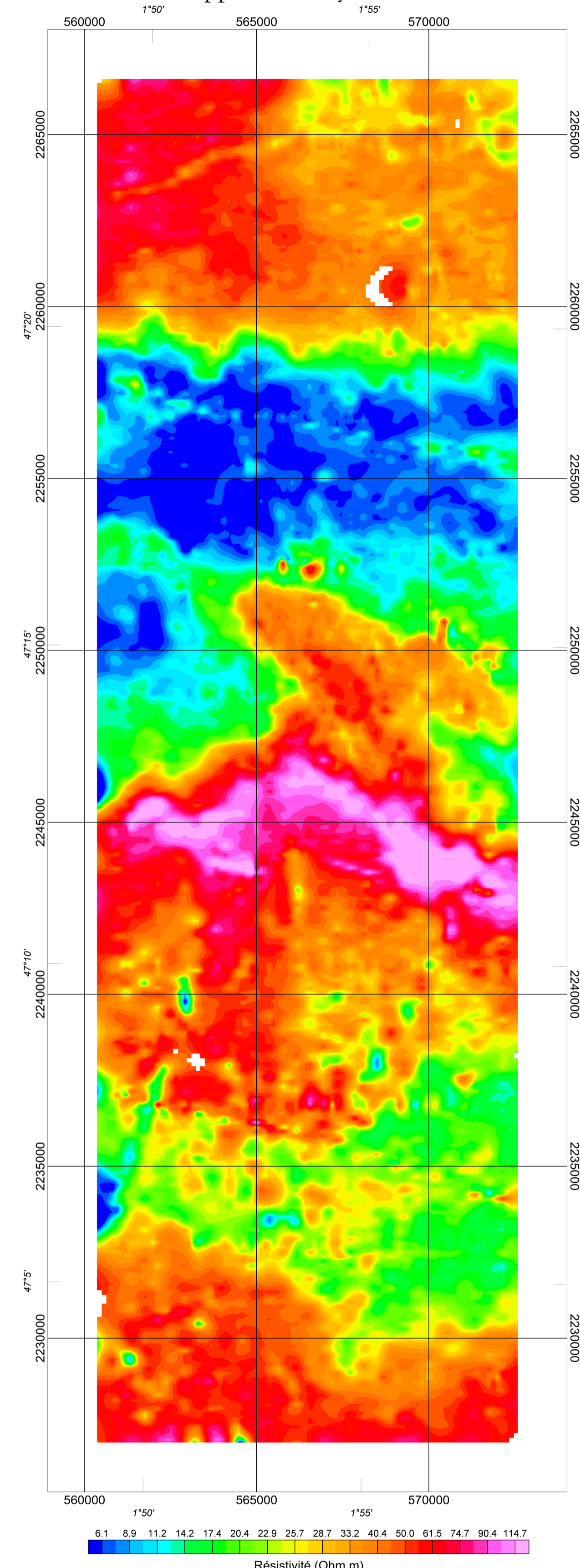
Résistivité apparente moyenne à 0/20 m
