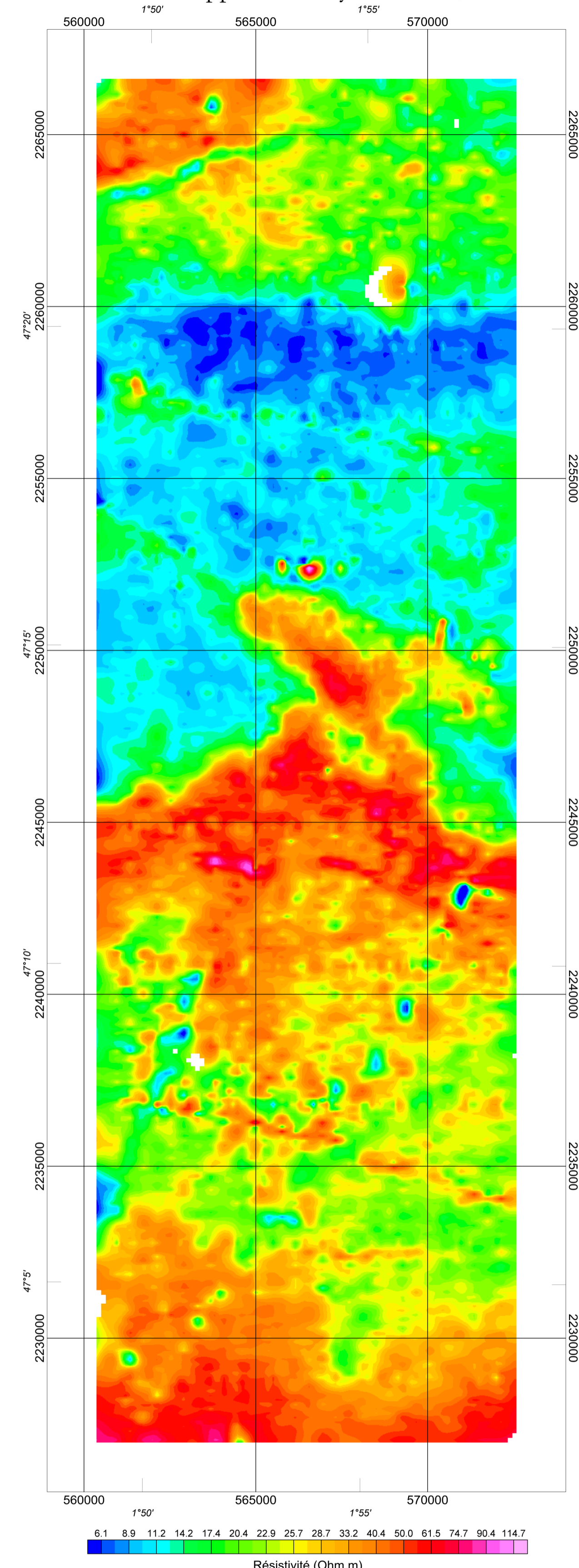
Résistivité apparente moyenne à -80/-60 m
